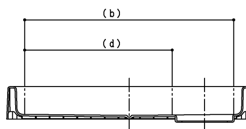
断面B-B
